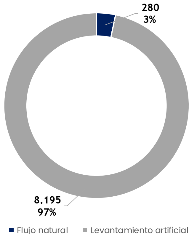
Mecanismo de producción por pozo
