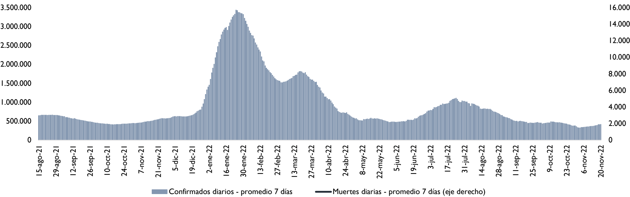
Casos diarios de COVID-19 en el mundo
